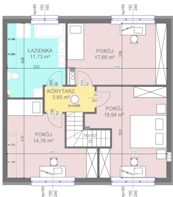
RZUT PIĘTRA
