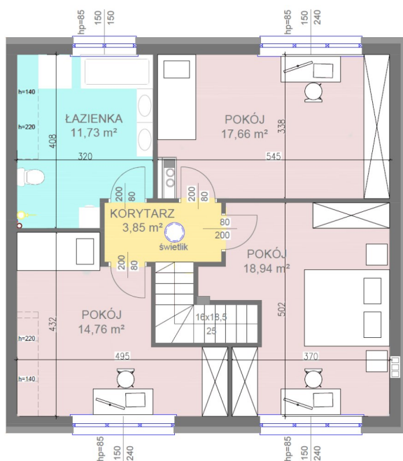
RZUT PIĘTRA
